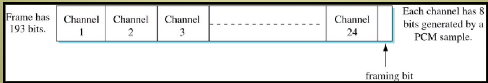
DS1 Frame
