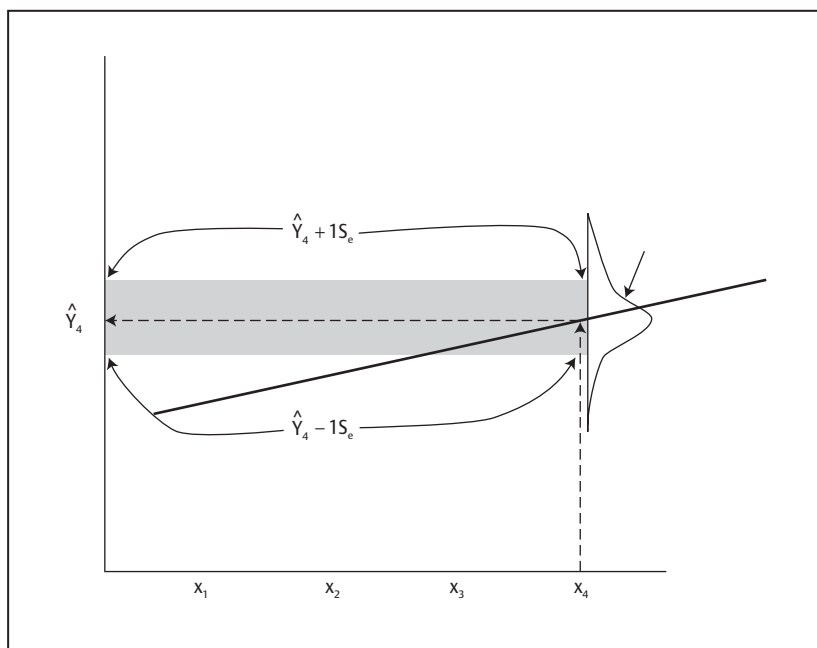
FIGURE 7.6 Représentation et utilisation de l'erreur type d'estimation pour les relations XY qui ne sont pas parfaites
