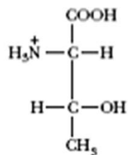
L-Threonine
