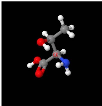
D-threonine
