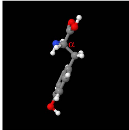
L-tyrosine
